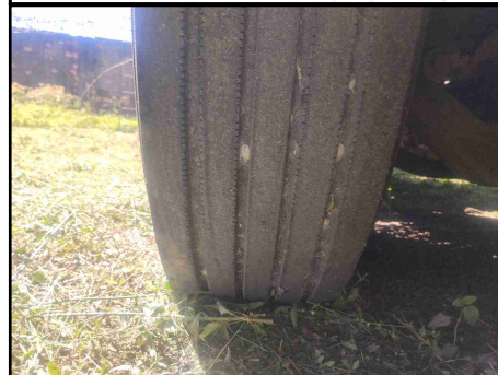
PNEU-RODA DIANTEIRO PASSAGEIRO
